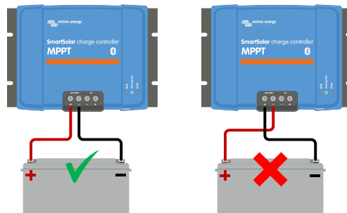
Beispiele für richtige und falsche (vertauschte) Batteriepolartät
