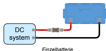
Einzelbatterie
