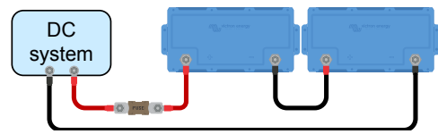
Mehrere Batterien in Reihe
