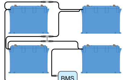
BMS-Anschluss für mehrere Batterien
