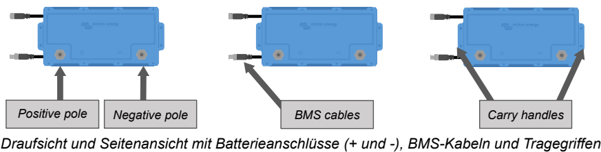
Draufsicht und Seitenansicht mit Batterieanschlüsse (+ und -), BMS-Kabeln und Tragegriffen
