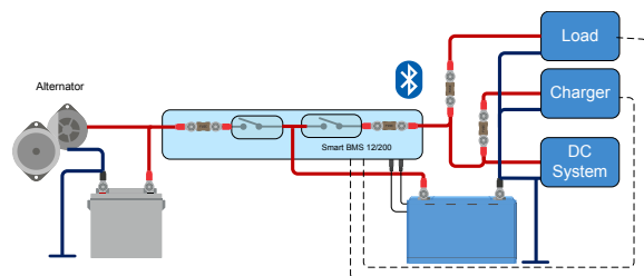
Das Smart BMS 12/200 steuert Lasten und Ladegeräte über die Signale „Lasttrennung“ und „Ladetrennung“. Es steuert und begrenzt auch die Lichtmaschine.
